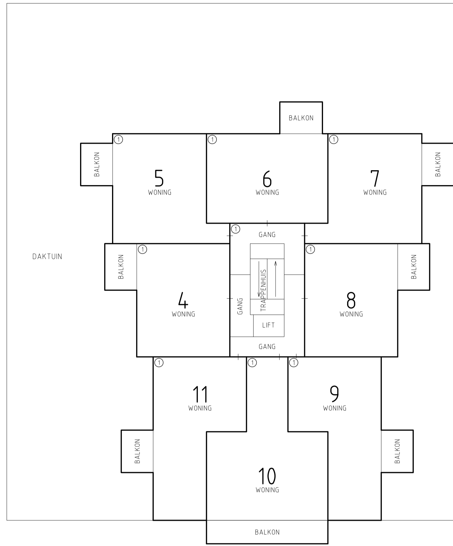
EERSTE ETAGE
