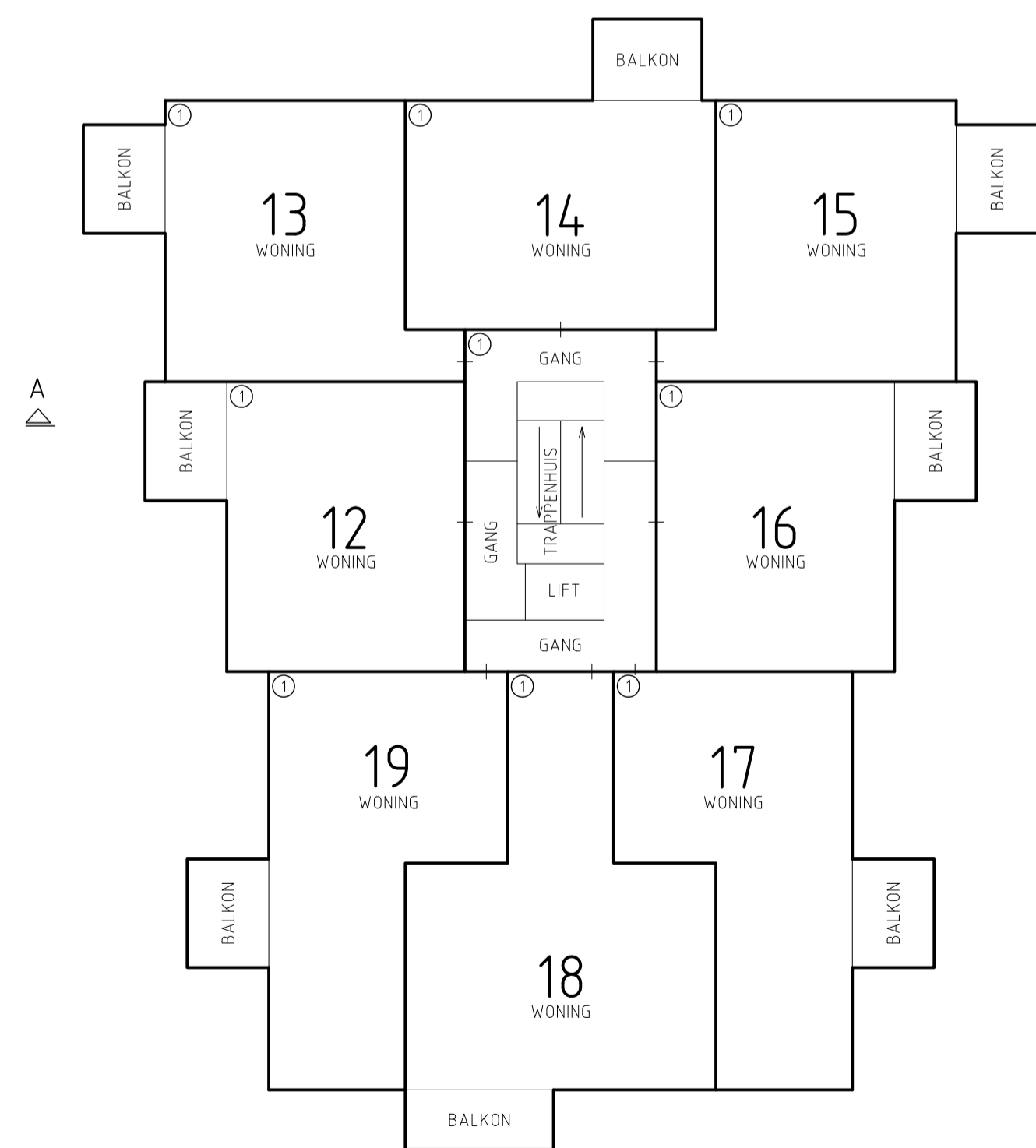
TWEDE ETAGE
